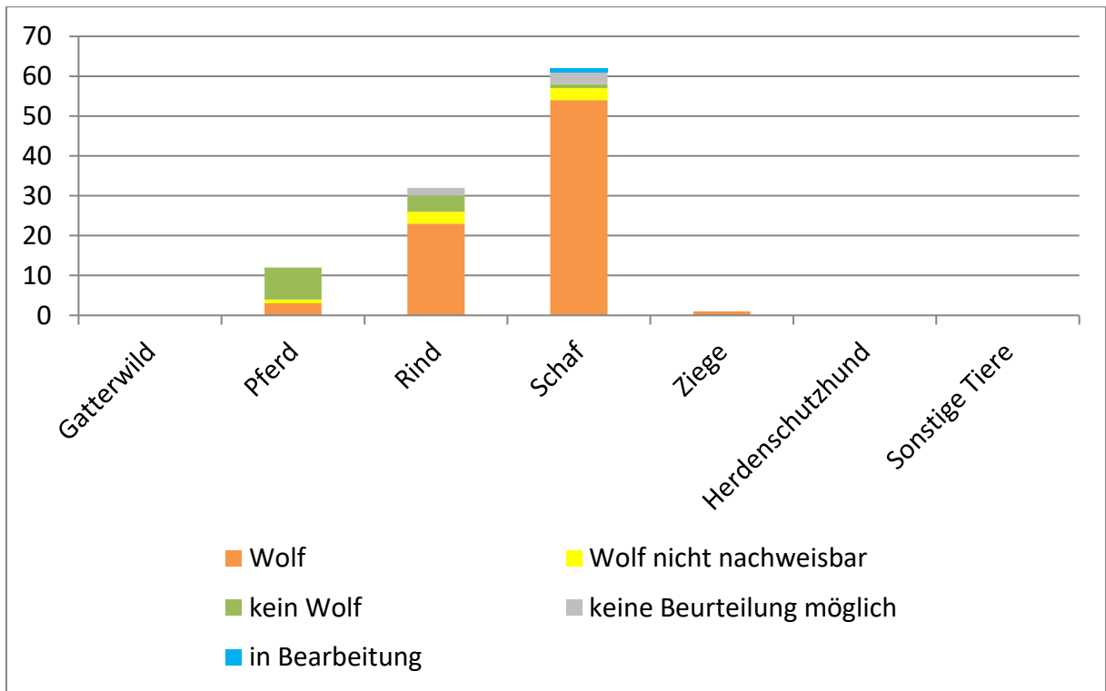
Abb. 24: Anzahl und amtliche Feststellung von Übergriffen auf unterschiedliche Tierarten im III. Quartal 2023 in Niedersachsen.
