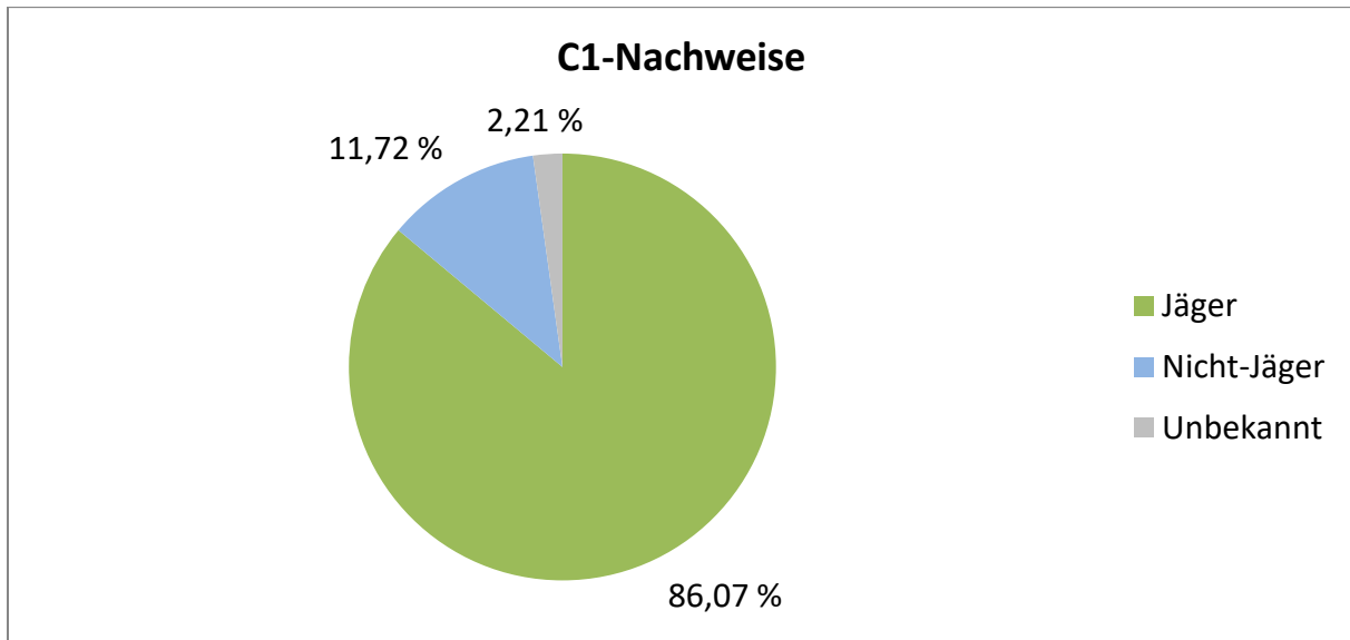
Abb. 9: Herkunft aller C1-Nachweise im III. Quartal 2023 an das Wolfsmonitoring nach Gruppenzugehörigkeit.
