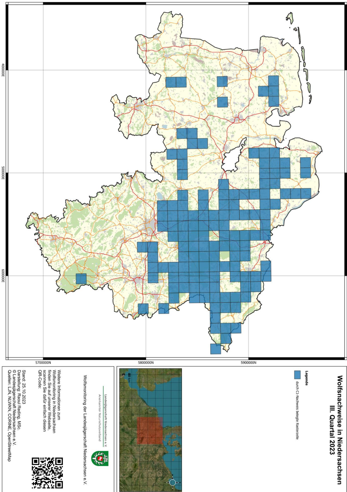
Abb. 21: Durch C1-Nachweise belegte Rasterzellen im EU-Grid 10 x 10km in Niedersachsen im III. Quartal 2023 (n=138).
