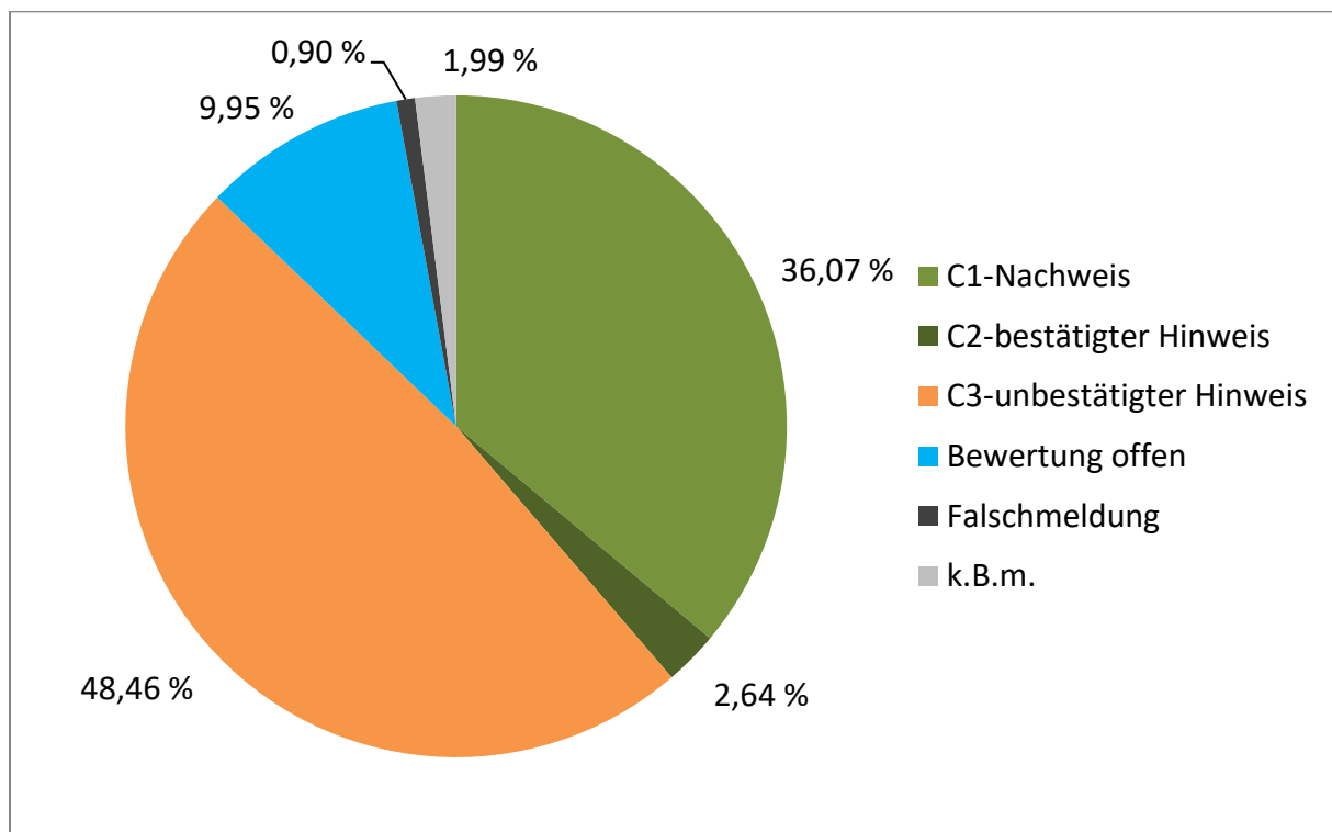
Abb. 5: Wolfsmeldungen im III. Quartal 2023 nach SCALP-Kriterium (n=2010).
