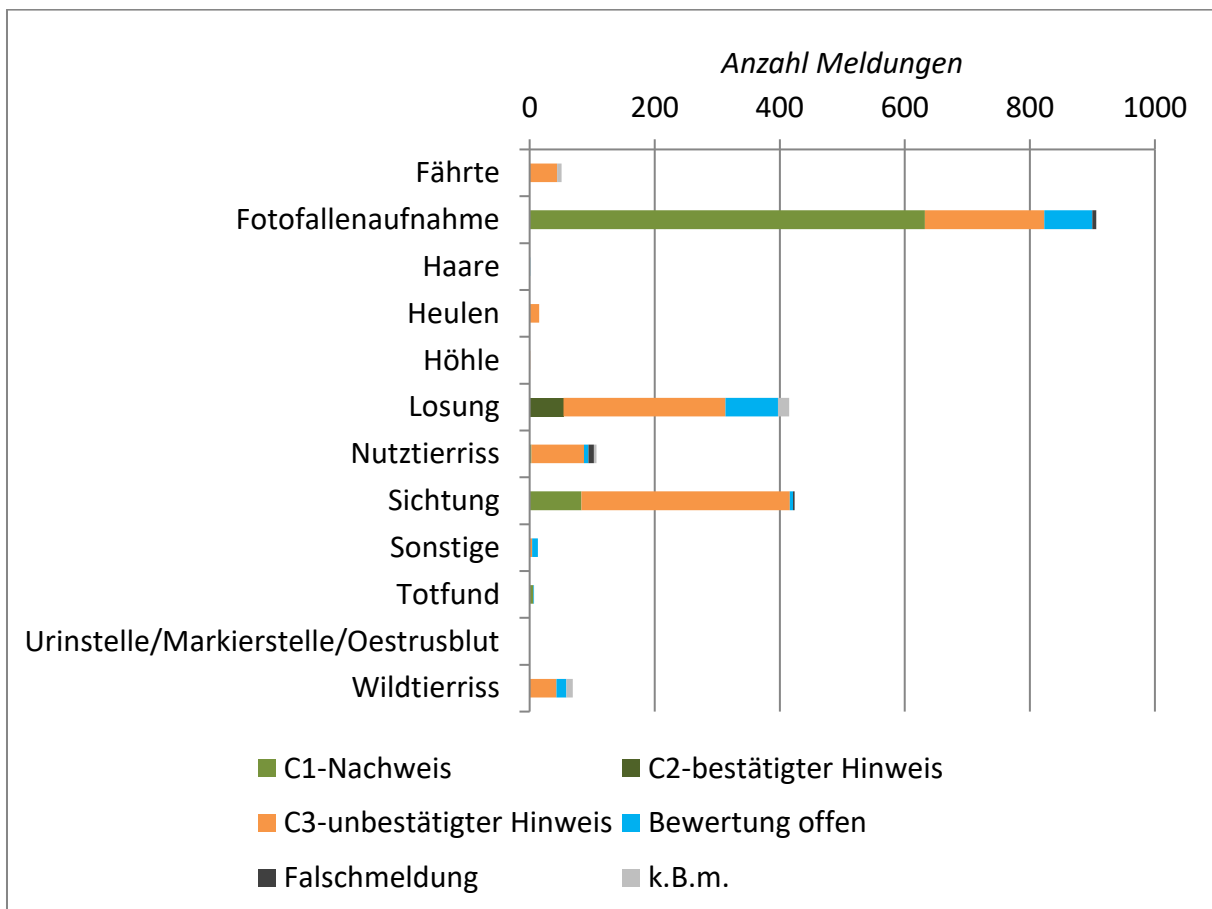
Abb. 6: Wolfsmeldungen im III. Quartal 2023 nach Meldungstyp und SCALP-Kriterium.
