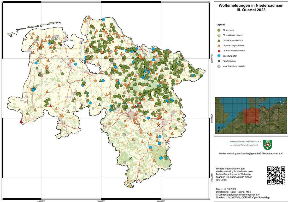
Abb. 19: Geografische Verteilung der Wolfsmeldungen im III. Quartal 2023 in Niedersachsen.
