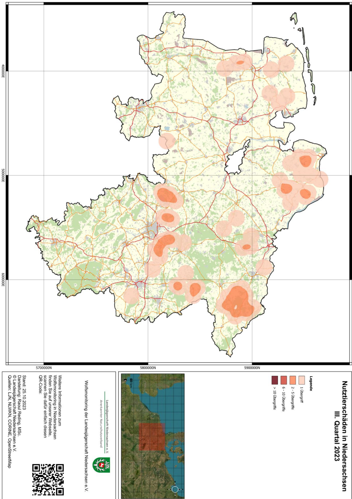
Abb. 27: Räumliche Dichte der durch den Wolf verursachten Nutztierschäden im III. Quartal 2023 in Niedersachsen.
