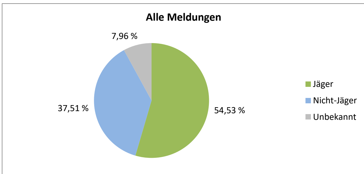
Abb. 8: Herkunft aller Meldungen im III. Quartal 2023 an das Wolfsmonitoring nach Gruppenzugehörigkeit.
