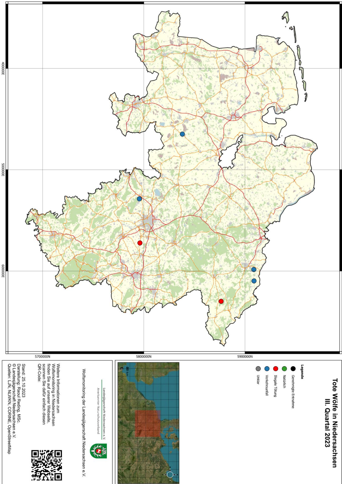
Abb. 23: Geografische Verteilung der Totfunde von Wölfen im III. Quartal 2023 in Niedersachsen.
