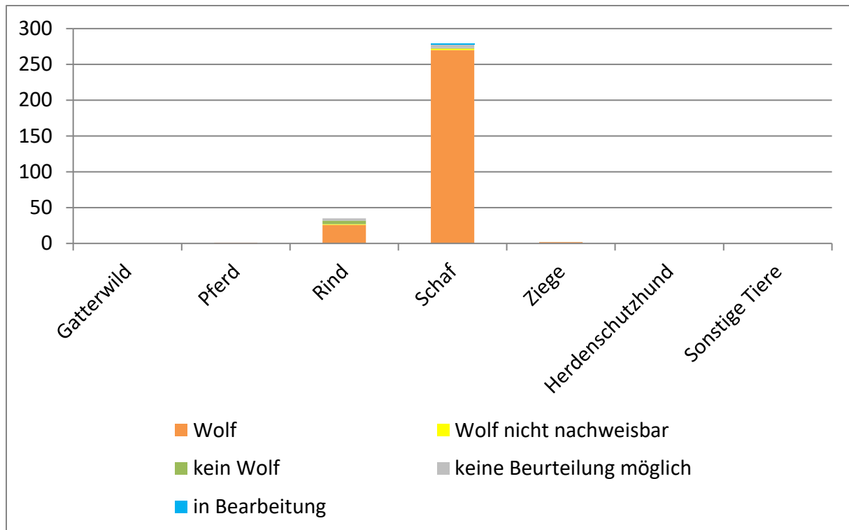
Abb. 25: Anzahl von getöteten Tieren im III. Quartal 2023 in Niedersachsen.
